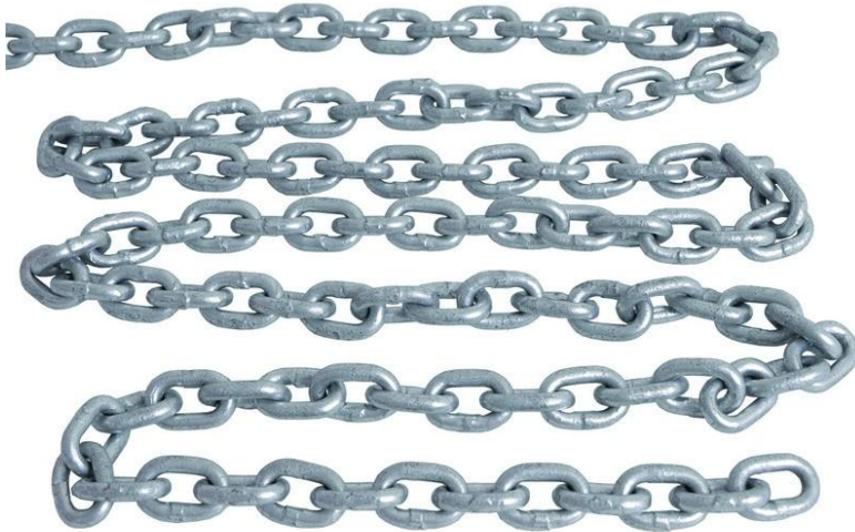
Galva chain Ø12 85m
